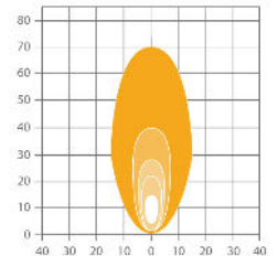
Long Range
