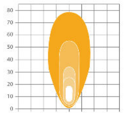
Long Range
