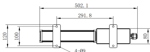
Modelo de montaje en pared (LY400-B-22W)
