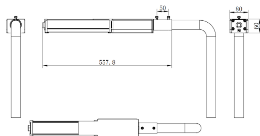
Modelo de montaje en poste (LY400-P-22W)
